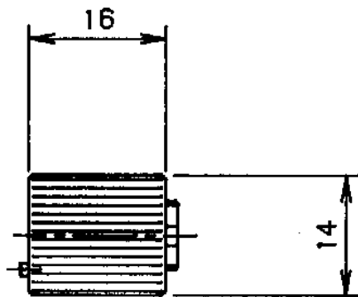
左側面图
